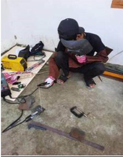
Gambar 2. Penyambungan pelat
